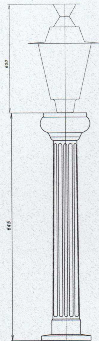
Градинско стълбче • Garden post
