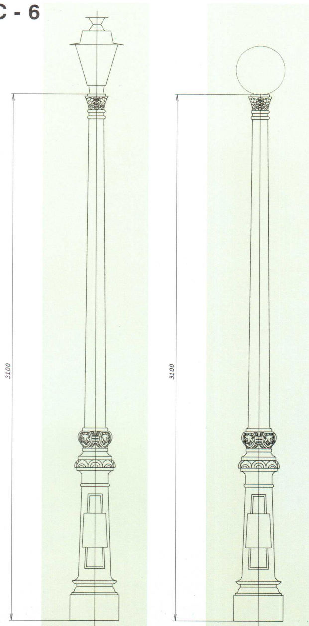
Осветителен стълб • Street lighting post
