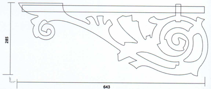
Стенна конзола • Wall brackets
